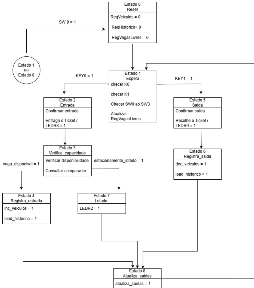
Figura 1 – Diagrama da FSM.
