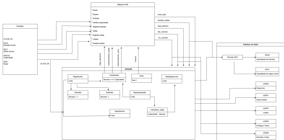
Figura 2 – Arquitetura RTL do Sistema.
